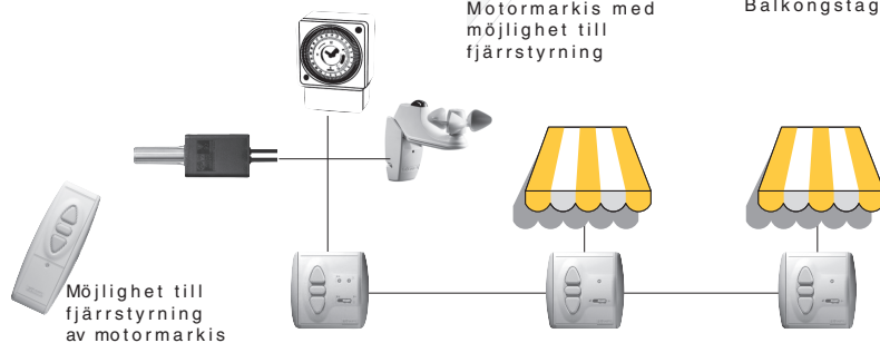
Sol och vindautomatik för flera motorer
