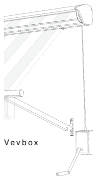
Snäckväxel / vev
