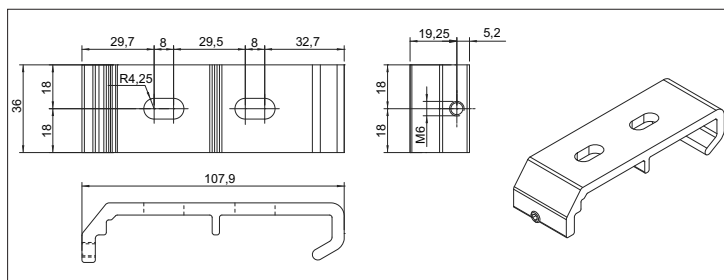
Väggbeslag Regent
