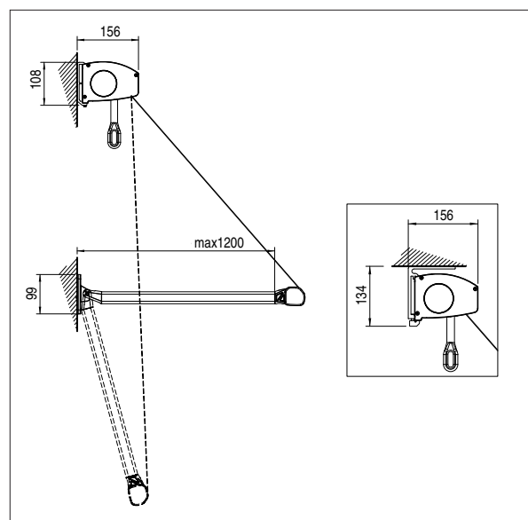
Måttsskiss Regent
