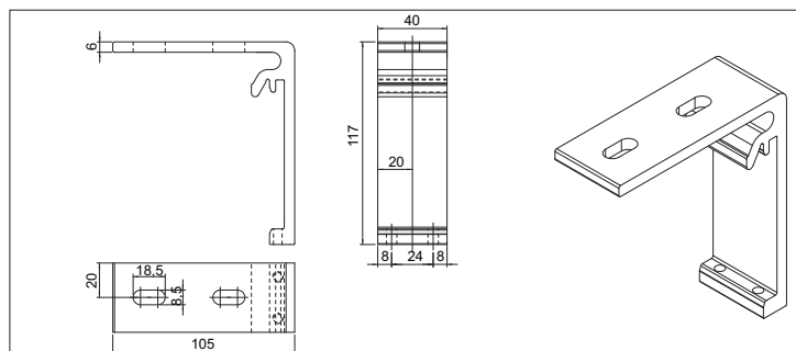
Takbeslag Regent
